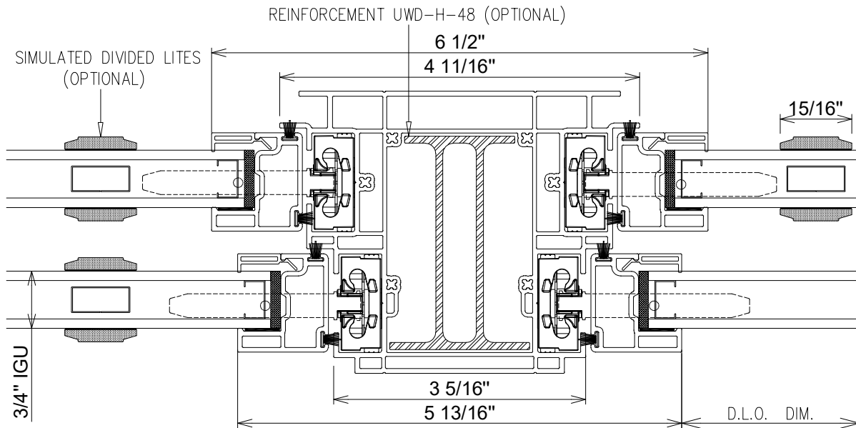
5 COMMON JAMB SECTION 5900 Scale: N.T.S.
