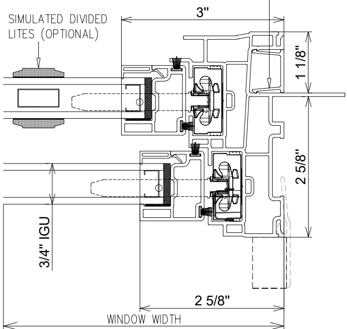
4 OPP JAMB SECTION
