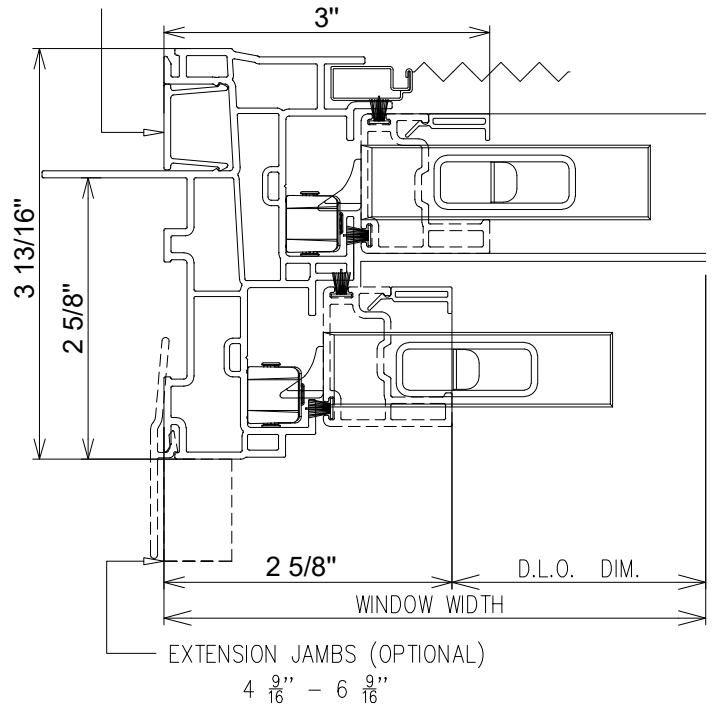
4 JAMB SECTION
