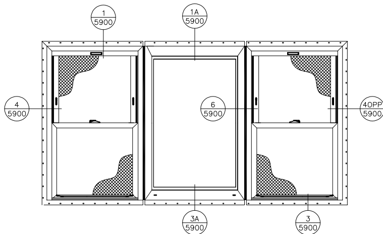
5900 DH - PW - DH
