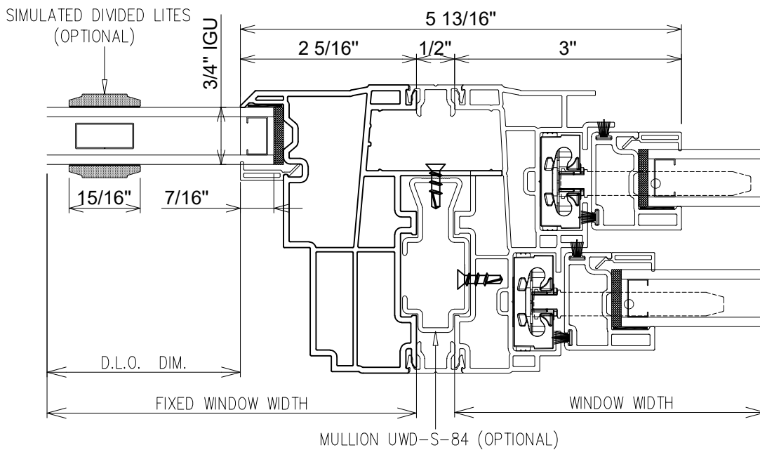
6 MULLION VERTICAL SECTION 5900 Scale: N.T.S.
